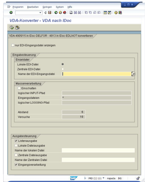
VDA nach IDoc im alogis-VDA-Konverter
